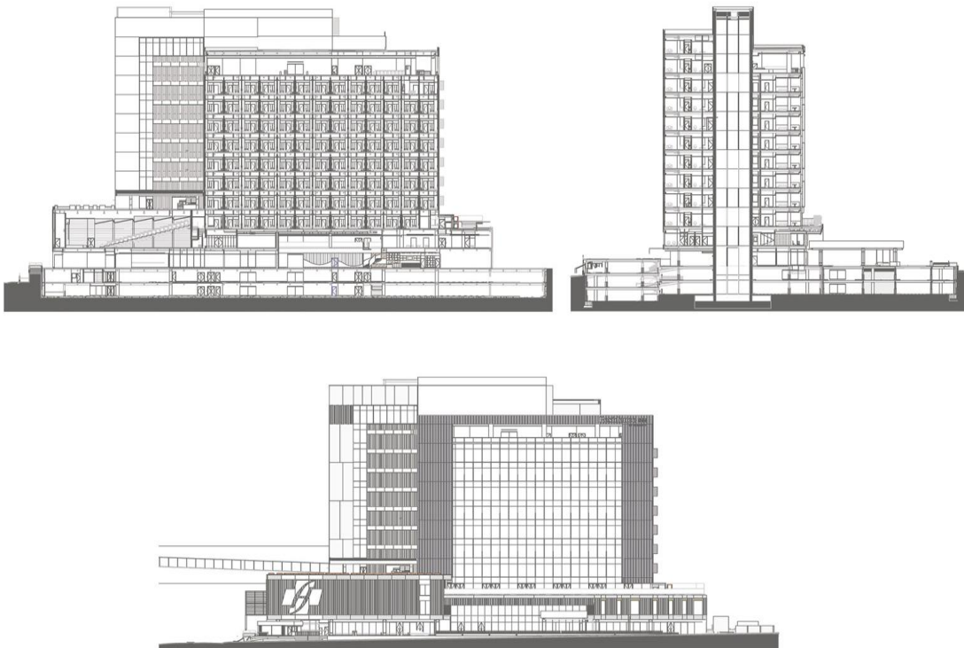
Secciones longitudinal y transversal y elevación frontal
